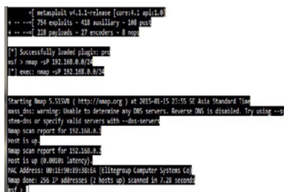
Gambar 4 Scanning IP yang aktif menggunakan Nmap
