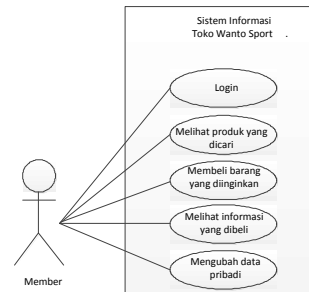
Gambar 2. Use Case untuk aktor Member
