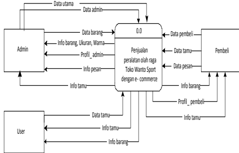
Gambar 4. Diagram Konteks
