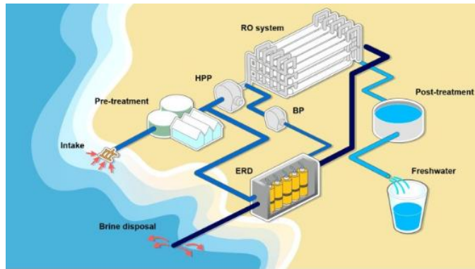
Sistem Sea Water Reverse Osmosis (SWRO) Sumber : Analisis Penulis, 2026
