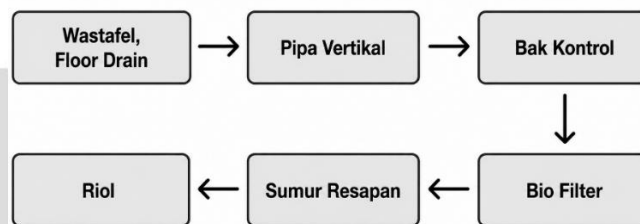
Sistem Utilitas Grey Water Sumber : Analisis Penulis, 2026
