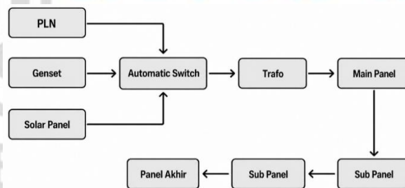
Sistem Utilitas Elektrikal Sumber : Analisis Penulis, 2026
