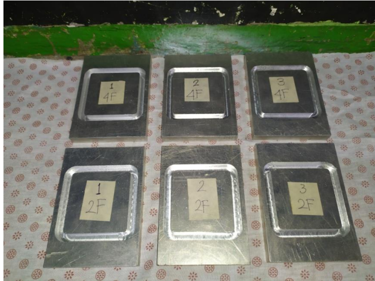
Lampiran 5. Spesimen Uji (Alumunium 5052)
