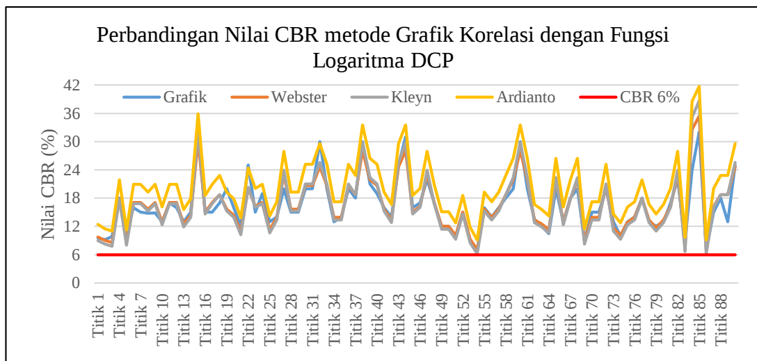
Gambar 2. Grafik perbandingan nilai CBR metode grafik korelasi dengan fungsi logaritma DCP
