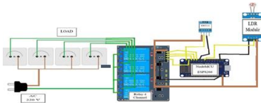
Gambar 3. Skematik Rangkaian
