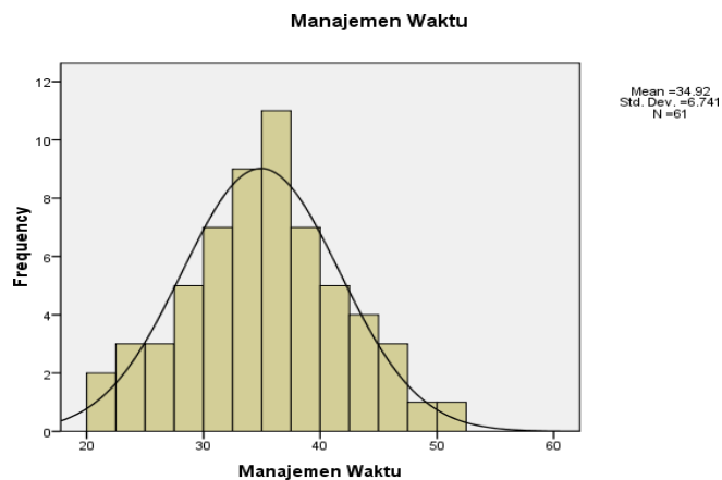
Gambar 2. Histogram dan Poligon Data Manajemen Waktu ( X_2 )
