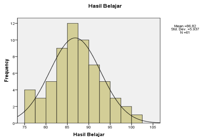
Gambar 3. Histogram dan Poligon Hasil Belajar (Y)
