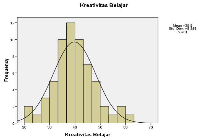
Gambar 1. Histogram dan Poligon Data Kreativitas Belajar ( X_1 )
