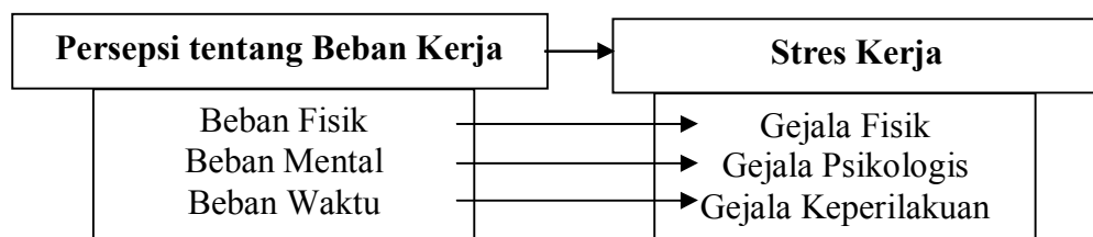
Gambar 1. Bagan Hubungan Persepsi tentang Beban Kerja terhadap Stres Kerja
