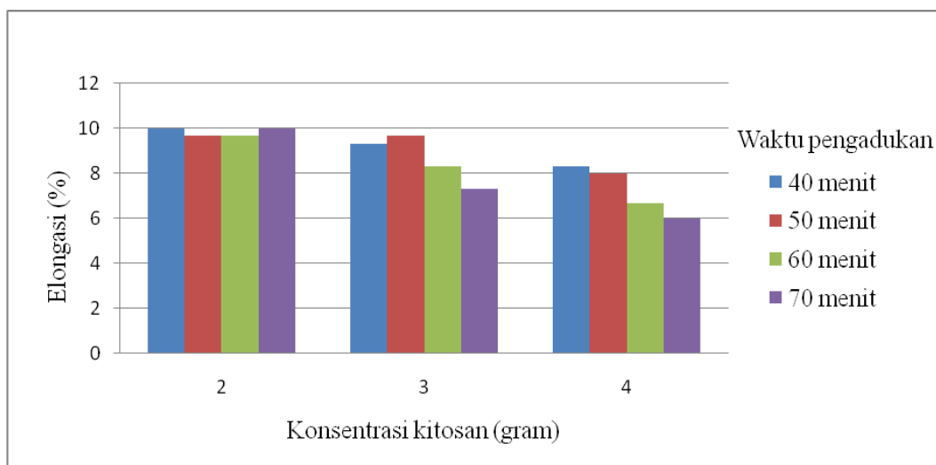
Gambar 3. Hasil rata-rata uji elongasi bioplastik
