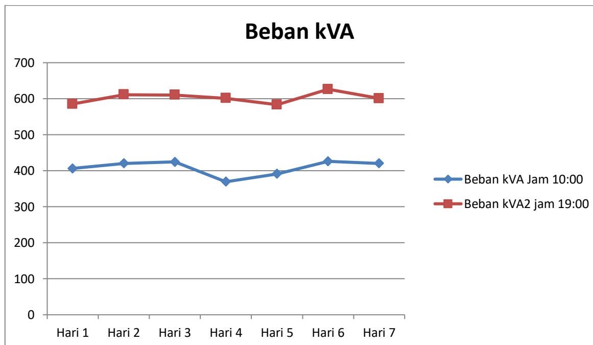
Gambar 2. Grafik pemakaian beban Transformator Unindo selama 7 hari
