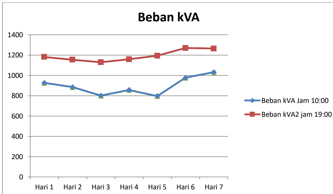
Gambar 2. Grafik pemakaian beban Transformator Starlite selama 7 hari
