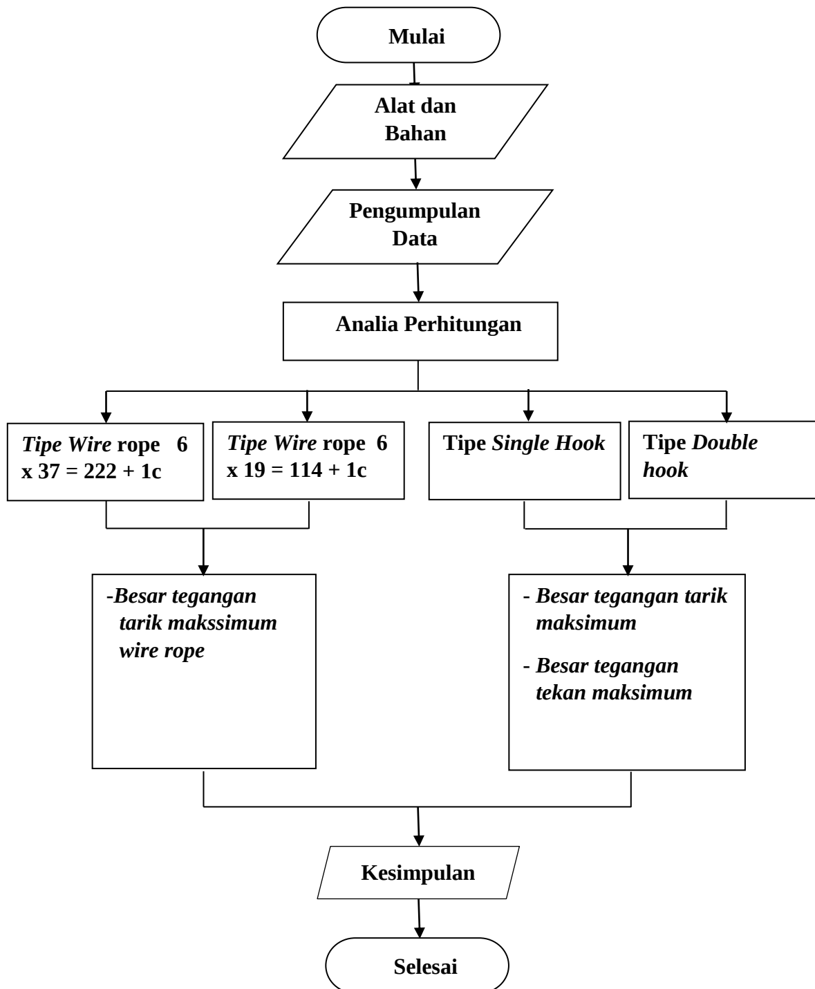
Gambar 3. Diagram alir pehitungan tengangan wire rope dan hook
