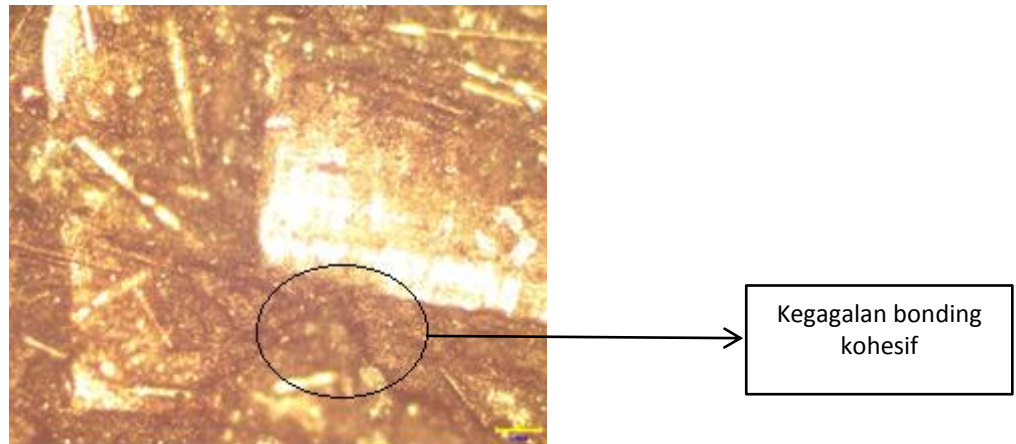
Gambar 12 Foto Mikro dengan variasi tembaga mesh 60 dan alumunium mesh 50 pembesaran 100x
