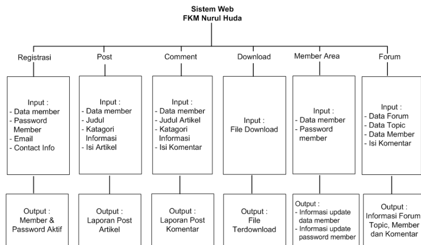
Gambar 4.2. Dekomposisi Proses Sistem Informasi Web FKM NH
