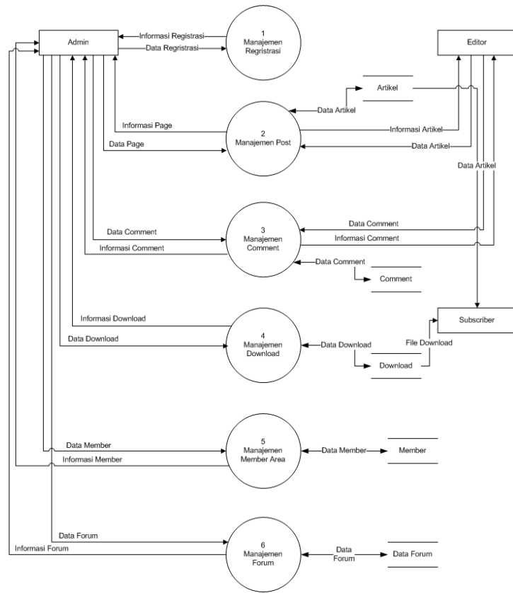
Gambar 4.3. Data Flow Diagram Sistem Informasi Web FKM NH
