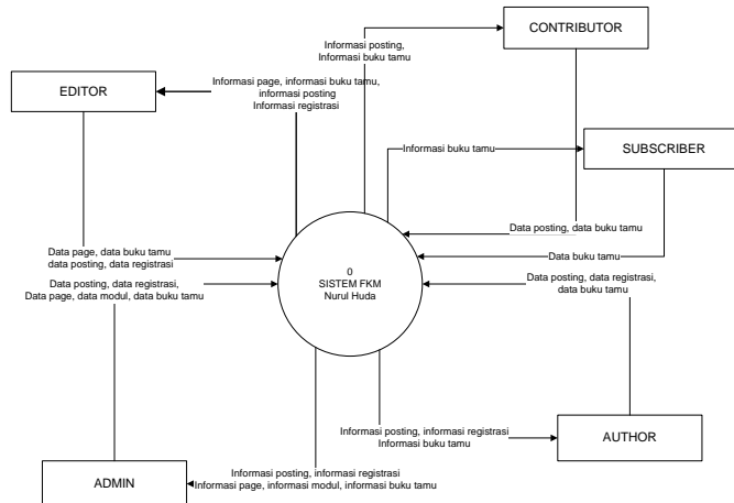
Gambar 4.1. Context Diagram Sistem Informasi Web FKM
