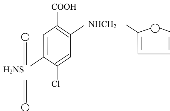
Gambar 2. Struktur Kimia Furosemida
