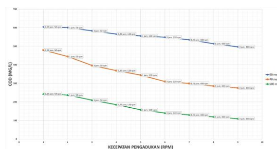
Gambar 1. Grafik COD
